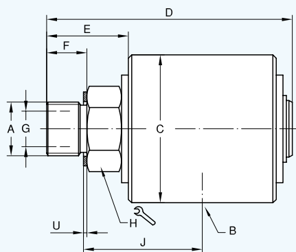
Одноточное ротационное соединение
