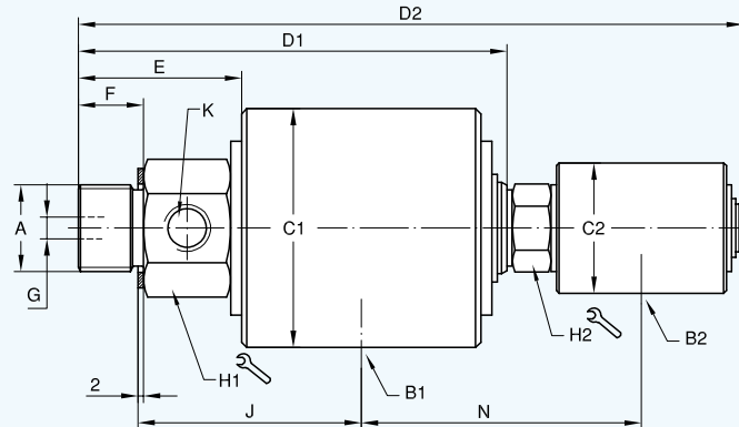
Двухточное ротационное соединение (тандем)
